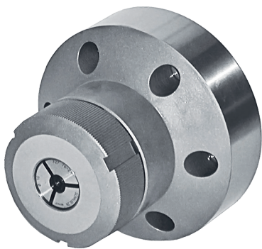
Kraftbetätigtes Druckspannzangenfutter F27
